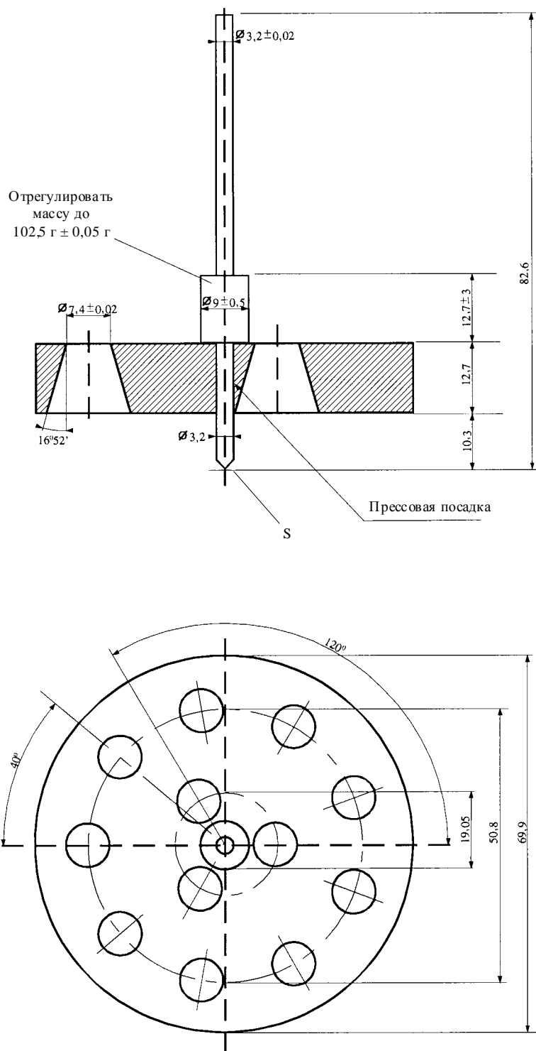
Рис. 1: Пенетрометр
